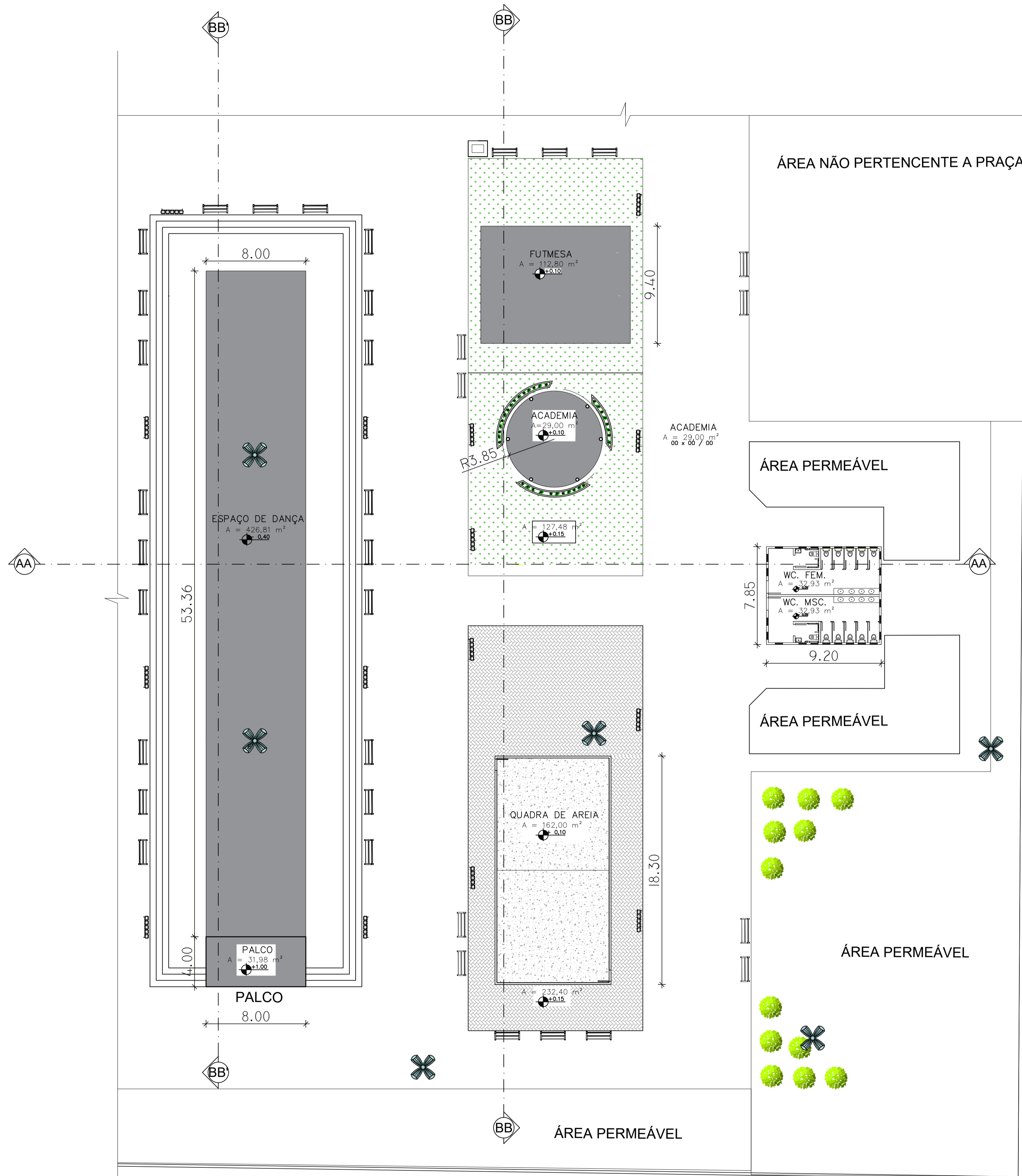
PRAÇA DA JUVENTUDE Planta Baixa de Piso Esc.1/200
